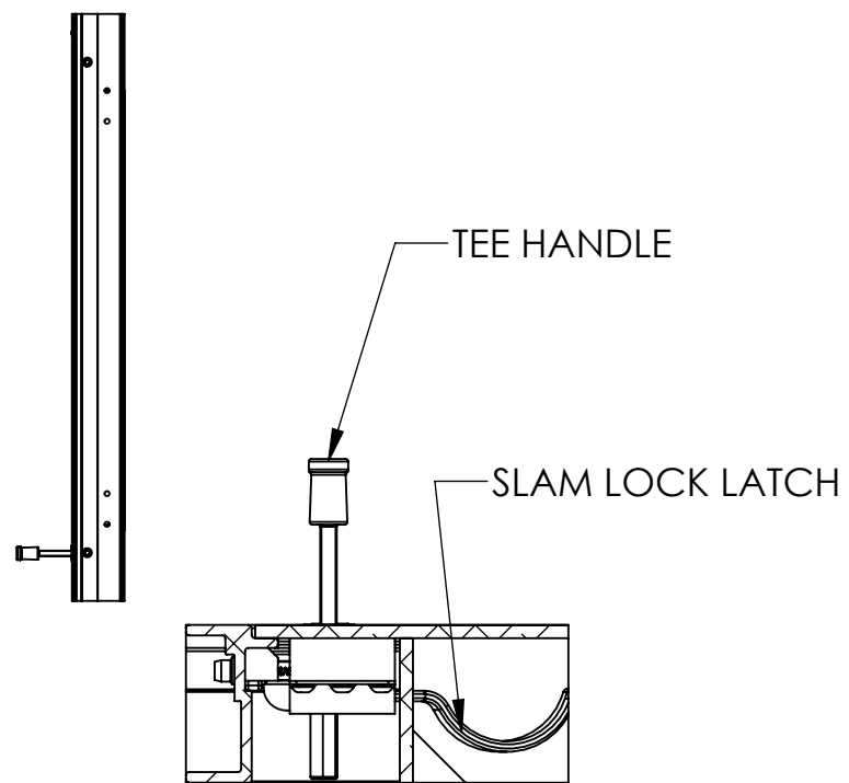
SECTION G-G SCALE 1 : 4
