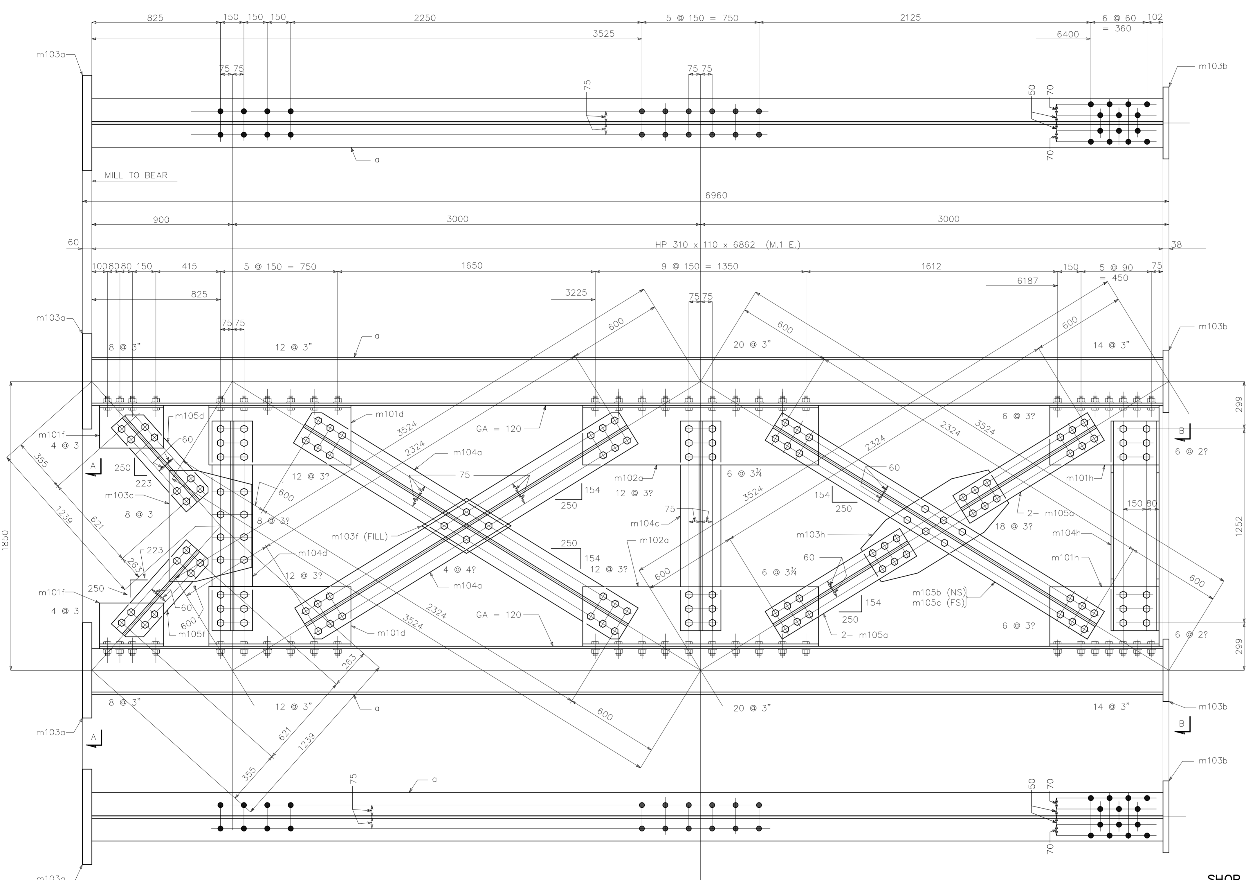
BENT ASSEMBLY MK. B3C
